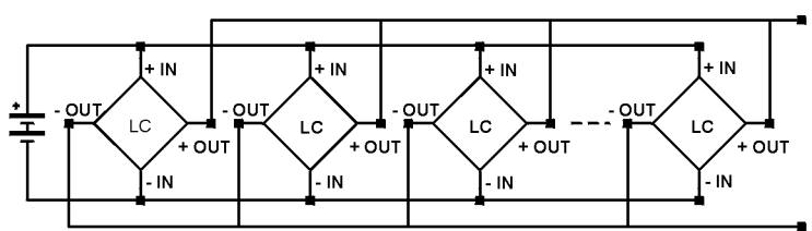
RACCORDEMENT 4 CELLULES OU PLUS EN PARALLELE
