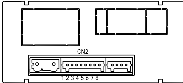
COMPTEUR MAGNÉTIQUE
