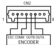
ENCODER
