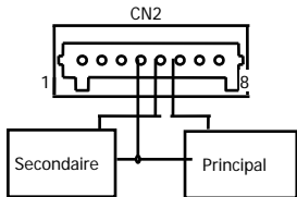
CAPTEUR NAMUR
