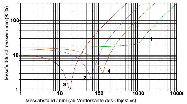
KT19.41 (3.9 \mu\text{m} ) KT19.21 (3.4 \mu\text{m} ) Detektor B Linse \text{CaF}_2 1 Objektiv K7 2 Objektiv L7 3 Objektiv M7 4 Objektiv N7
