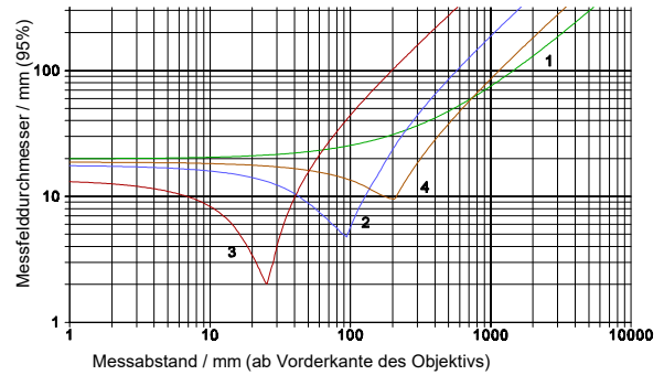
KT19.43 (7.5 ... 8.2 µm) Detektor A Linse CaF 2 1 Objektiv K7 2 Objektiv L7 3 Objektiv M7 4 Objektiv N7
