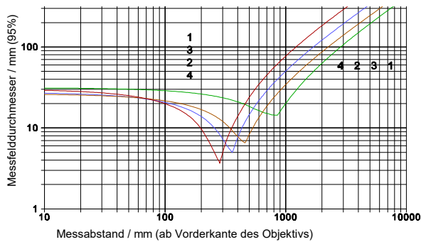
KT19.41 (3.9 \mu\text{m} ) KT19.21 (3.4 \mu\text{m} ) Detektor B Objektiv S922 Linse \text{CaF}_2 1 ohne Zwischenring 2 mit Zwischenring 1 3 mit Zwischenring 2 4 mit Zwischenring 1+2
