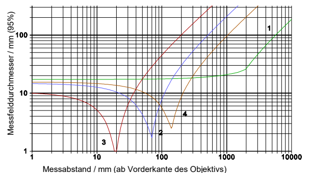
KT19.42 (4.9 ... 5.5 \mu\text{m} ) Detektor C Linse \text{CaF}_2 1 Objektiv K7 2 Objektiv L7 3 Objektiv M7 4 Objektiv N7
