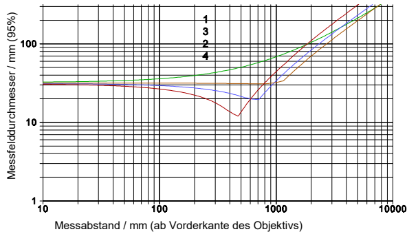
KT19.43 (7.5 ... 8.2 µm) Detektor A Objektiv S922 Linse CaF 2 1 ohne Zwischenring 2 mit Zwischenring 1 3 mit Zwischenring 2 4 mit Zwischenring 1+2
