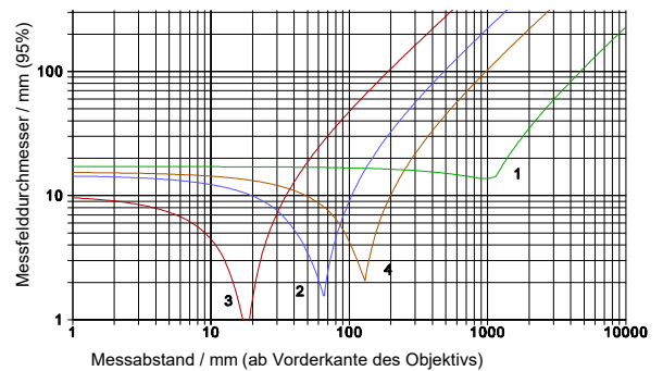
KT19.41 (3.9 \mu\text{m} ) KT19.21 (3.4 \mu\text{m} ) Detektor C Linse \text{CaF}_2 1 Objektiv K7 2 Objektiv L7 3 Objektiv M7 4 Objektiv N7
