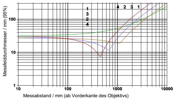
KT19.43 (7.5 ... 8.2 µm) Detektor B Objektiv S922 Linse CaF 2 1 ohne Zwischenring 2 mit Zwischenring 1 3 mit Zwischenring 2 4 mit Zwischenring 1+2
