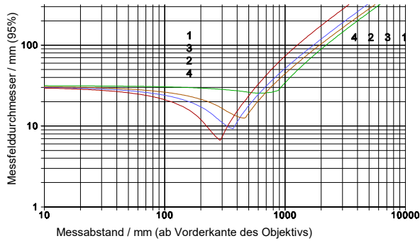
KT19.41 (3.9 \mu\text{m} ) KT19.21 (3.4 \mu\text{m} ) Detektor A Objektiv S922 Linse \text{CaF}_2 1 ohne Zwischenring 2 mit Zwischenring 1 3 mit Zwischenring 2 4 mit Zwischenring 1+2
