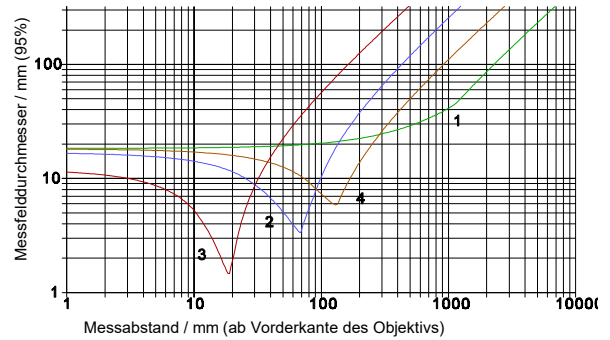
KT19.41 (3.9 \mu\text{m} ) KT19.21 (3.4 \mu\text{m} ) Detektor A Linse \text{CaF}_2 1 Objektiv K7 2 Objektiv L7 3 Objektiv M7 4 Objektiv N7
