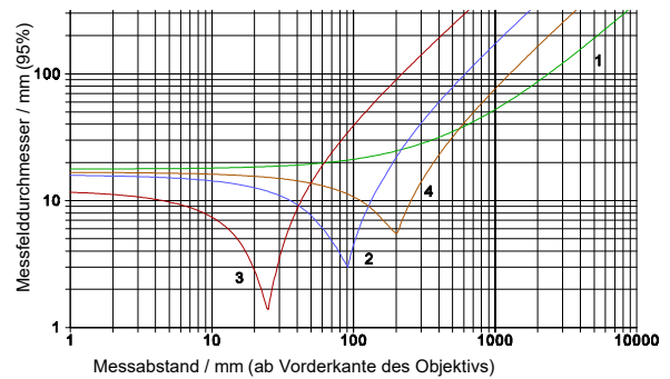
KT19.43 (7.5 ... 8.2 µm) Detektor B Linse CaF 2 1 Objektiv K7 2 Objektiv L7 3 Objektiv M7 4 Objektiv N7
