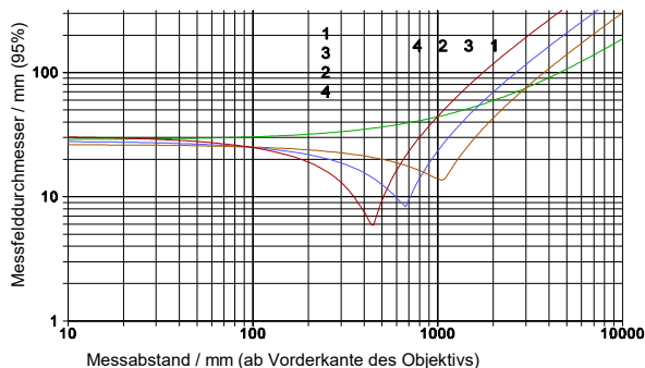
KT19.43 (7.5 ... 8.2 µm) Detektor C Objektiv S922 Linse CaF 2 1 ohne Zwischenring 2 mit Zwischenring 1 3 mit Zwischenring 2 4 mit Zwischenring 1+2
