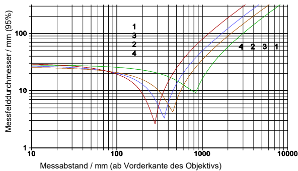
KT19.41 (3.9 \mu\text{m} ) KT19.21 (3.4 \mu\text{m} ) Detektor C Objektiv S922 Linse \text{CaF}_2 1 ohne Zwischenring 2 mit Zwischenring 1 3 mit Zwischenring 2 4 mit Zwischenring 1+2
