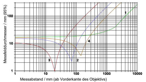
KT19.42 (4.9 ... 5.5 \mu\text{m} ) Detektor B Linse \text{CaF}_2 1 Objektiv K7 2 Objektiv L7 3 Objektiv M7 4 Objektiv N7
