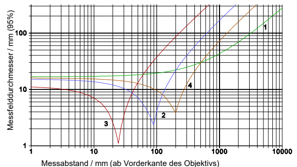
KT19.43 (7.5 ... 8.2 µm) Detektor C Linse CaF 2 1 Objektiv K7 2 Objektiv L7 3 Objektiv M7 4 Objektiv N7
