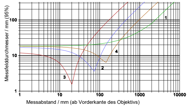
KT19.42 (4.9 ... 5.5 \mu\text{m} ) Detektor A Linse \text{CaF}_2 1 Objektiv K7 2 Objektiv L7 3 Objektiv M7 4 Objektiv N7
