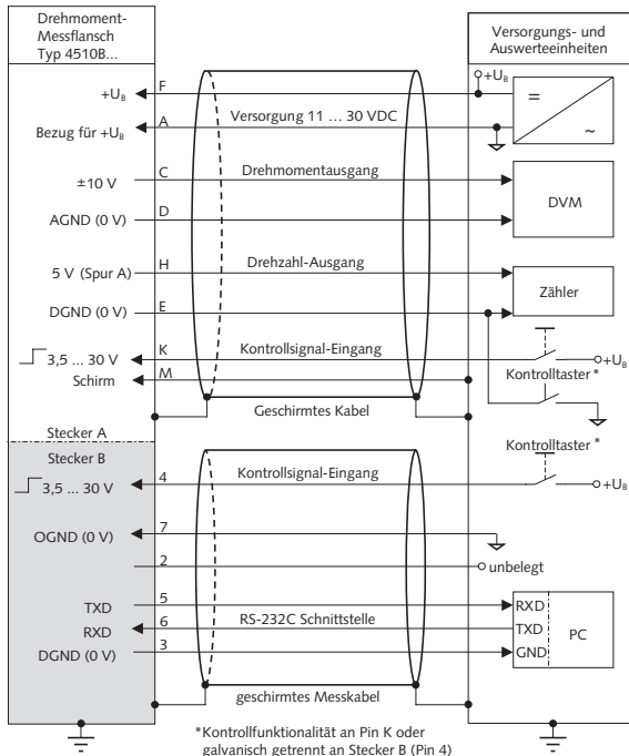
Bild 5: Anschlusschema des Einbaustecker A und B (standard)
