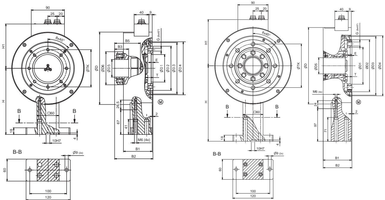
Bild 1: Typ 4510B... Baugrösse 1 und 3, 100 N·m, 200 N·m, 1 000 N·m, 2 000 N·m, 4 000 N·m
