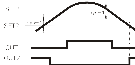
Asymmetrische Hysterese
