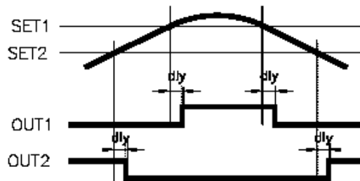
Zeitverzögerungsverhalten
