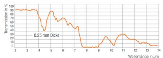
Spektrale Durchlässigkeit von Kunststofffolien aus Polyester
