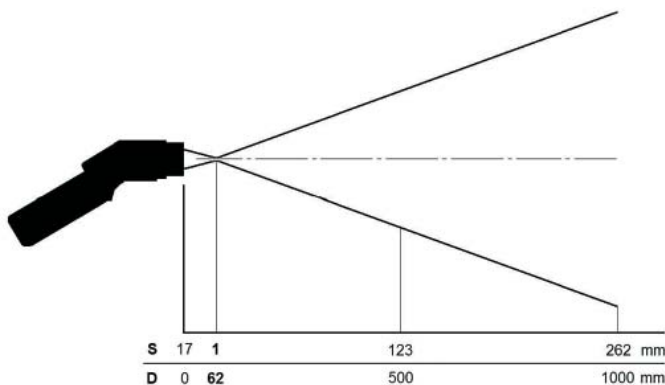
Optisches Diagramm einer Scharfunkt optik
