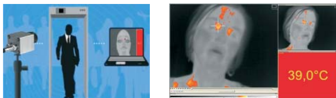
Anlage zum Hauttemperaturscreening an Reisenden mit Präzisionsreferenzstrahler
