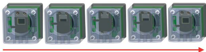
Zur Offsetreferenzierung wird das Gesichtsfeld des Infrarot-Sensorarrays mittels Linearmotor kurzzeitig geschlossen
