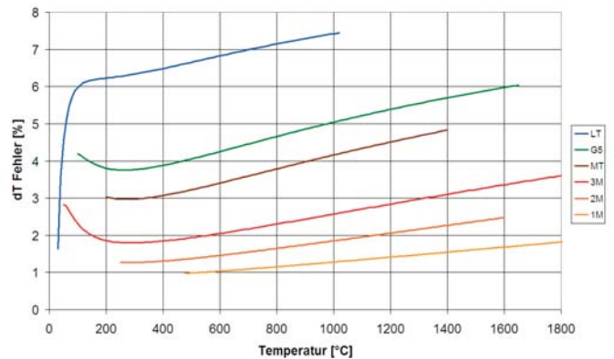
Messfehler bei 10 Prozent falsch eingestelltem Emissionsgrad in Abhängigkeit von der Wellenlänge und Objekttemperatur (LT: 8-14 \mu\text{m} ; G5: 5 \mu\text{m} ; MT: 3,9 \mu\text{m} ; 3M: 2,3 \mu\text{m} ; 2M: 1,6 \mu\text{m} ; 1M: 1,0 \mu\text{m} ).
