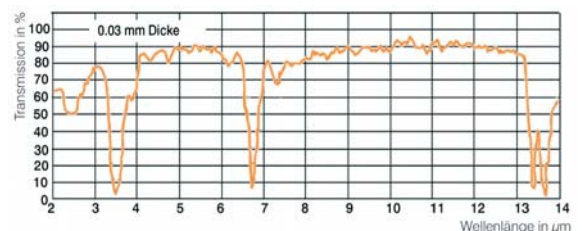
Spektrale Durchlässigkeit von Kunststofffolien aus Polyäthylen
