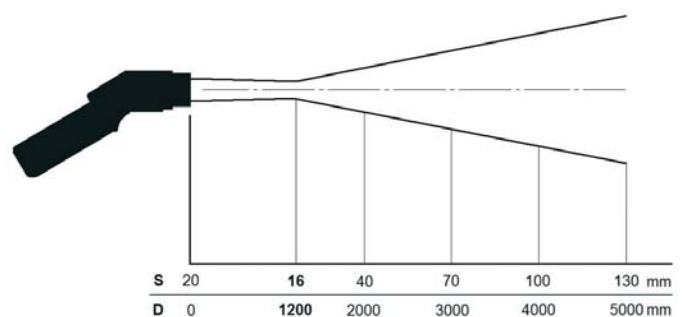
Optisches Diagramm eines Infrarotsensors
