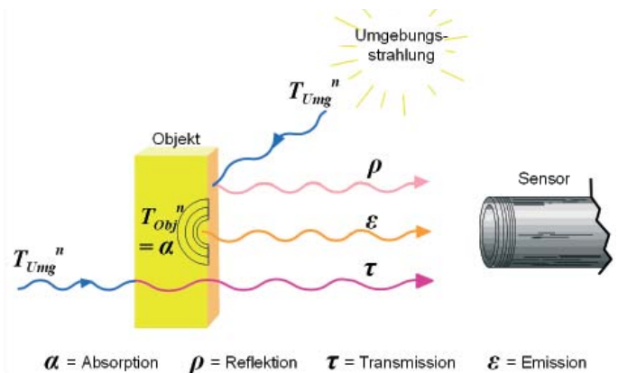
Umgebungsstrahlungskompensation
