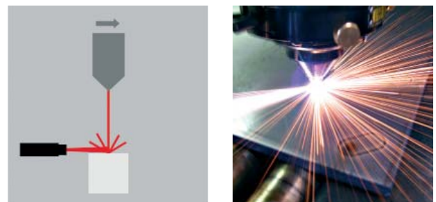
Infrarottemperaturmessung beim Laserschweißen
