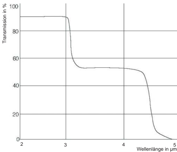
Spektraler Durchlässigkeit von Glas
