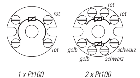
Kennzeichnung Keramiksockel bei 4-Leiterschaltung
