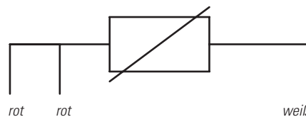
Schaltbild 3-Leiterschaltung
